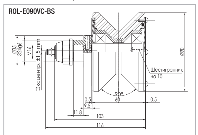
Максимальная нагрузка: в радиальном направлении 1150 Н, в осевом направлении 650 Н. Опция: смазка на весь срок службы. Рис. 106
