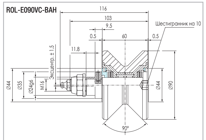
Воздействие нагрузки в радиальном направлении: не более 1150 Н. Рис. 104
