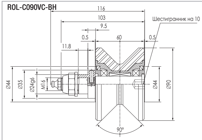
Максимальная нагрузка: в радиальном направлении 1150 Н, в осевом направлении 650 Н Рис. 101
