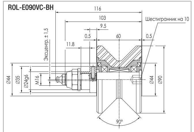
Максимальная нагрузка: в радиальном направлении 1150 Н, в осевом направлении 650 Н Рис. 102
