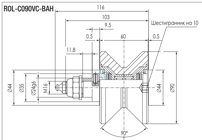
Воздействие нагрузки в радиальном направлении: не более 1150 Н. Рис. 103
