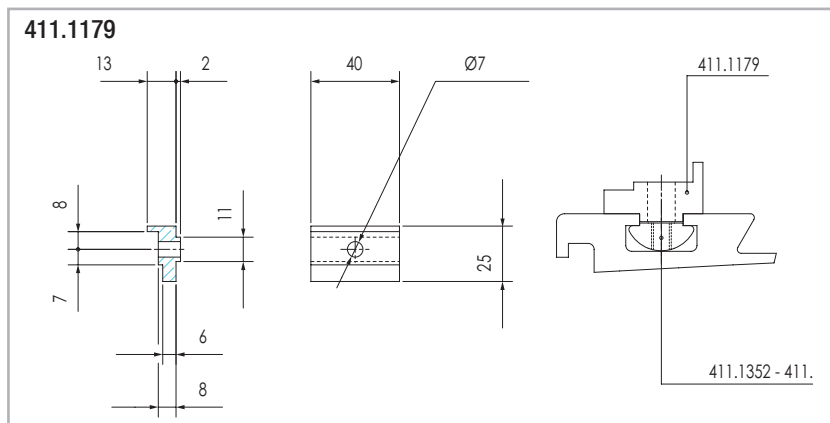
Модуль «2», прямой зуб
