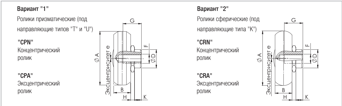
Уплотнения: резиновое "2RS", обеспечивающее брызгозащиту, или в виде стального защитного диска "2Z" (для типоразмера "63" стальной защитный диск идёт под кодом "2ZR"). Примечание: подшипники роликов заправлены заводской смазкой, рассчитанной на весь срок эксплуатации. Рис. 42
