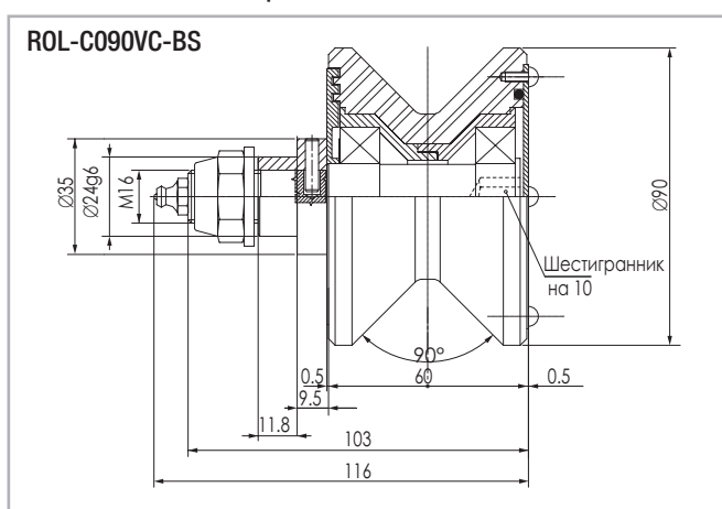
Максимальная нагрузка: в радиальном направлении 1150 Н, в осевом направлении 650 Н. Опция: смазка на весь срок службы. Рис. 105
